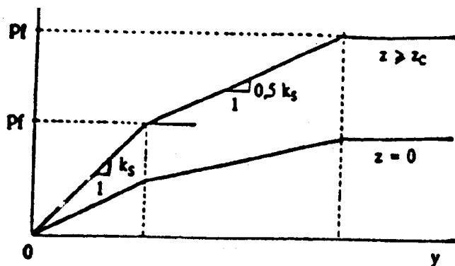
شکل شماره (۱۸-۴) - نمودار (P - Y) برای شمع با بار جانبی
