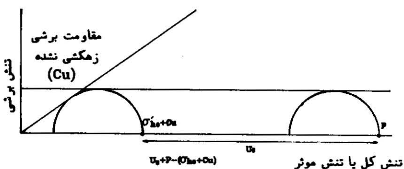
شکل شماره (۴-۹-ج) - پس از افزایش فشار درون گمانه
