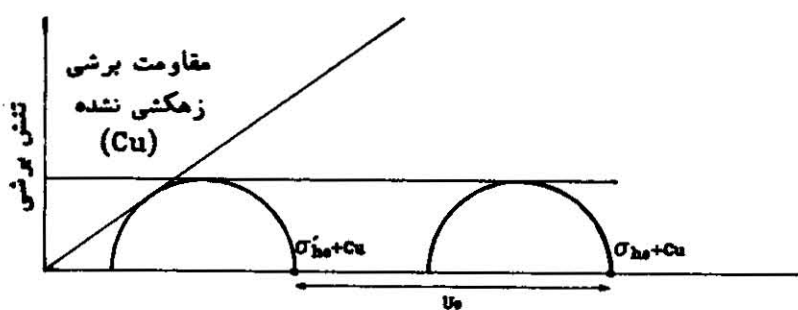
تنش کل یا تنش موثر شکل شماره (۴-۹-ب) - شروع تغییر شکل خمیری
