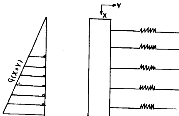
شکل (۱۹-۴) - شمع مدل شده با فنر
