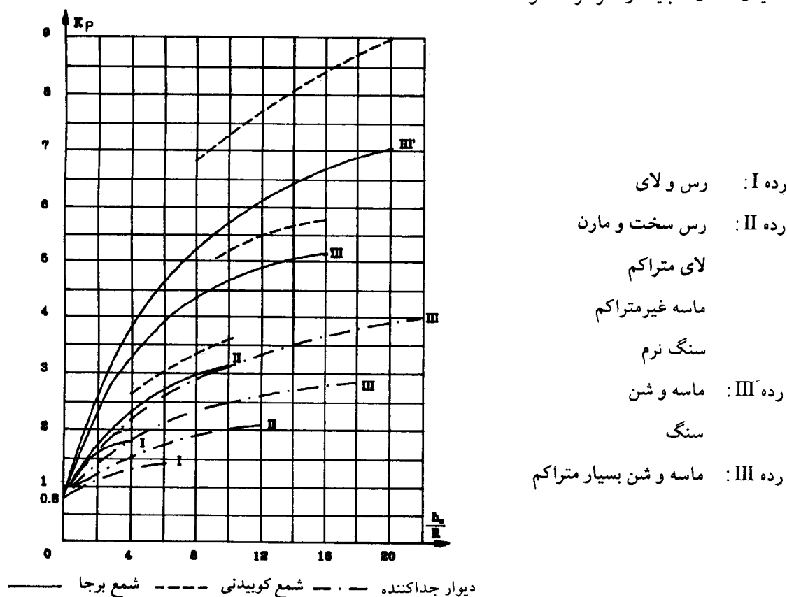
شکل شماره (۱۵-۴) - ضریب باربری پرسیمتر منارد M.P.M نوک شمع برای پی‌های عمیق ( k_p ) [۵-۱]
