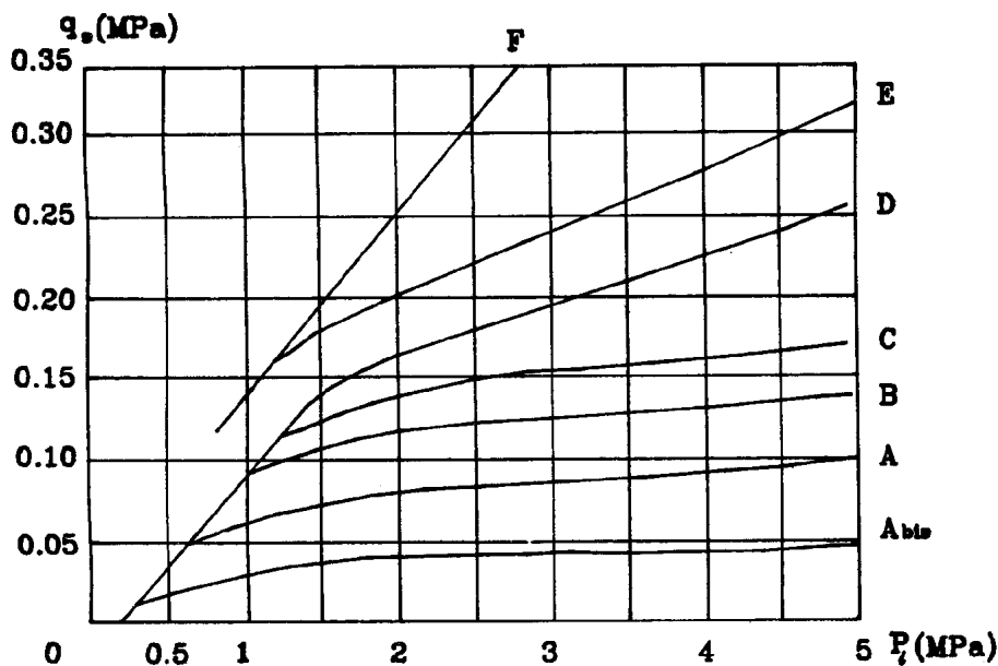
شکل شماره (۴-۱۶) - منحنی‌های P_u برحسب q_s برای انواع شمعها
