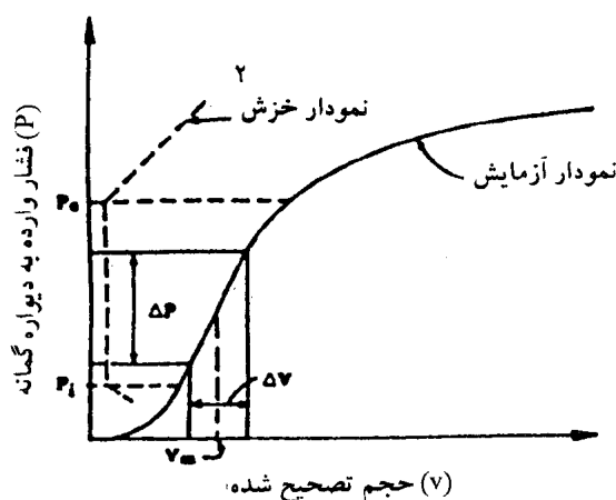
شکل شماره (۴-۱ ب) - نمودار پرسیومتري به روش (ب) V-P
