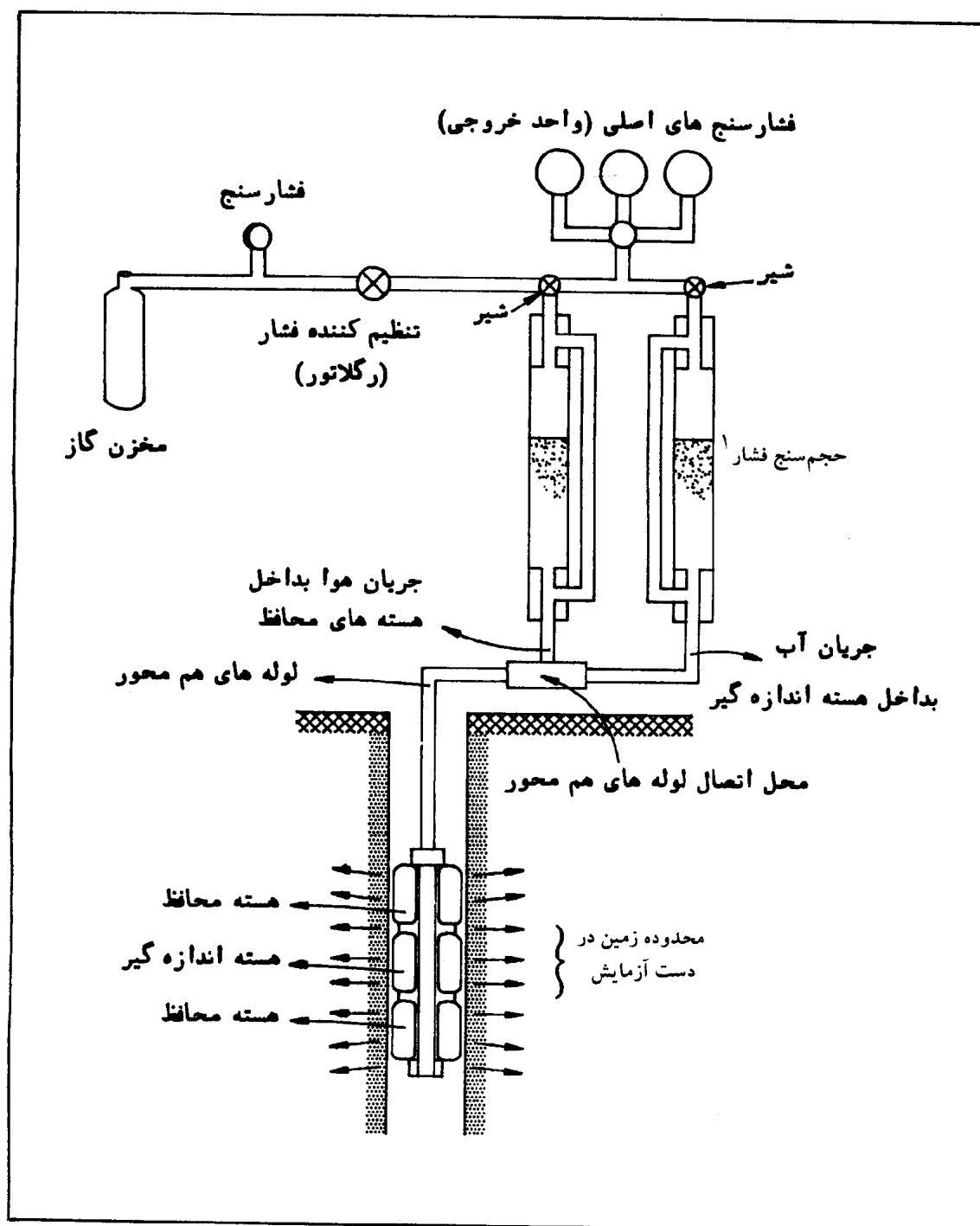
شکل شماره (۱-۱) - شمای دستگاه پرسومتر
