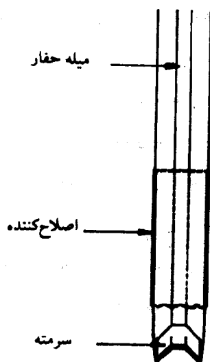
شکل شماره (۴-۳) - آماده سازی یک گمانه آزمایش با روش حفاری باگمانه پیشتاز و اصلاح همزمان
