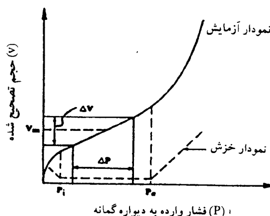
شکل شماره (۴-۱ الف) - نمودار پرسیومتري به روش (الف) P-V
